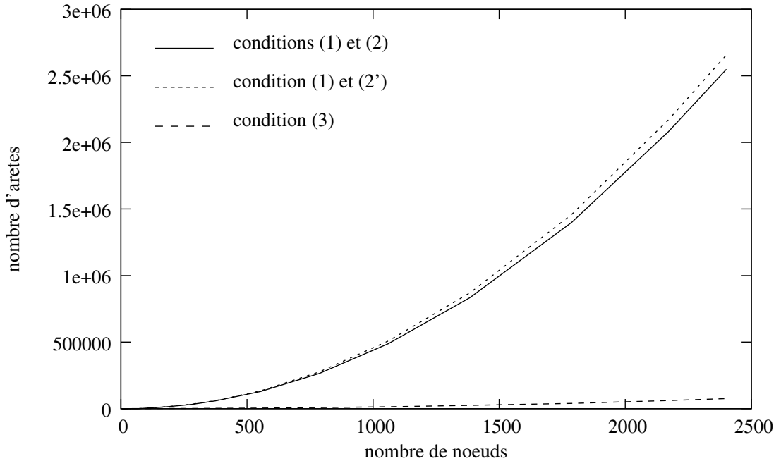
FIG. 3.11 – Nombre d'arêtes en fonction du nombre de nœuds dans les GC en utilisant soit les conditions (1) et (2), soit les conditions (1) et (2'), soit la condition (3).
